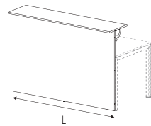
TBF12 L120 P40 H110,4 TBF14 L140 P40 H110,4 TBF16 L160 P40 H110,4 TBF18 L180 P40 H110,4 TBF20 L200 P40 H110,4
