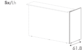
TBF7 L1,8 P61,8 H107,2 TBF6 L1,8 P61,8 H107,2
